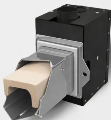
Palnik Platinum Bio 1 z nakładką ceramiczną
