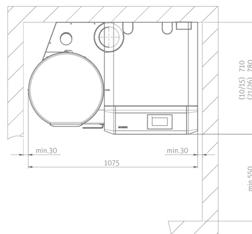
Widok z góry, minimalne odstępy: (podłączenie kominia z góry*)
